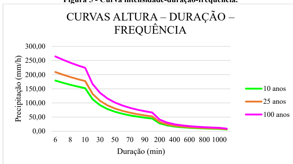
Figura 5 - Curva intensidade-duração-frequência.
